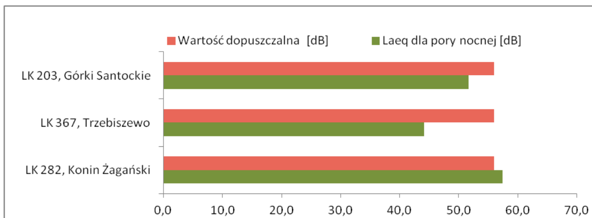
Rys. 42. Wartość zmierzonego poziomu dźwięku hałasu kolejowego dla pory nocnej w 2016 r. w porównaniu z wartością dopuszczalną
