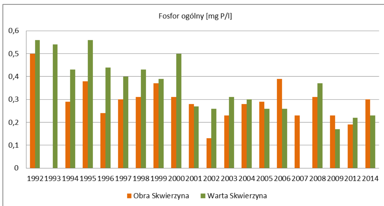
Rys. 10. Średnioroczne wartości stężenia fosforu ogólnego [mg P/l] w wybranych rzekach na terenie Skwierzyzny badanych w latach 1992-2014
