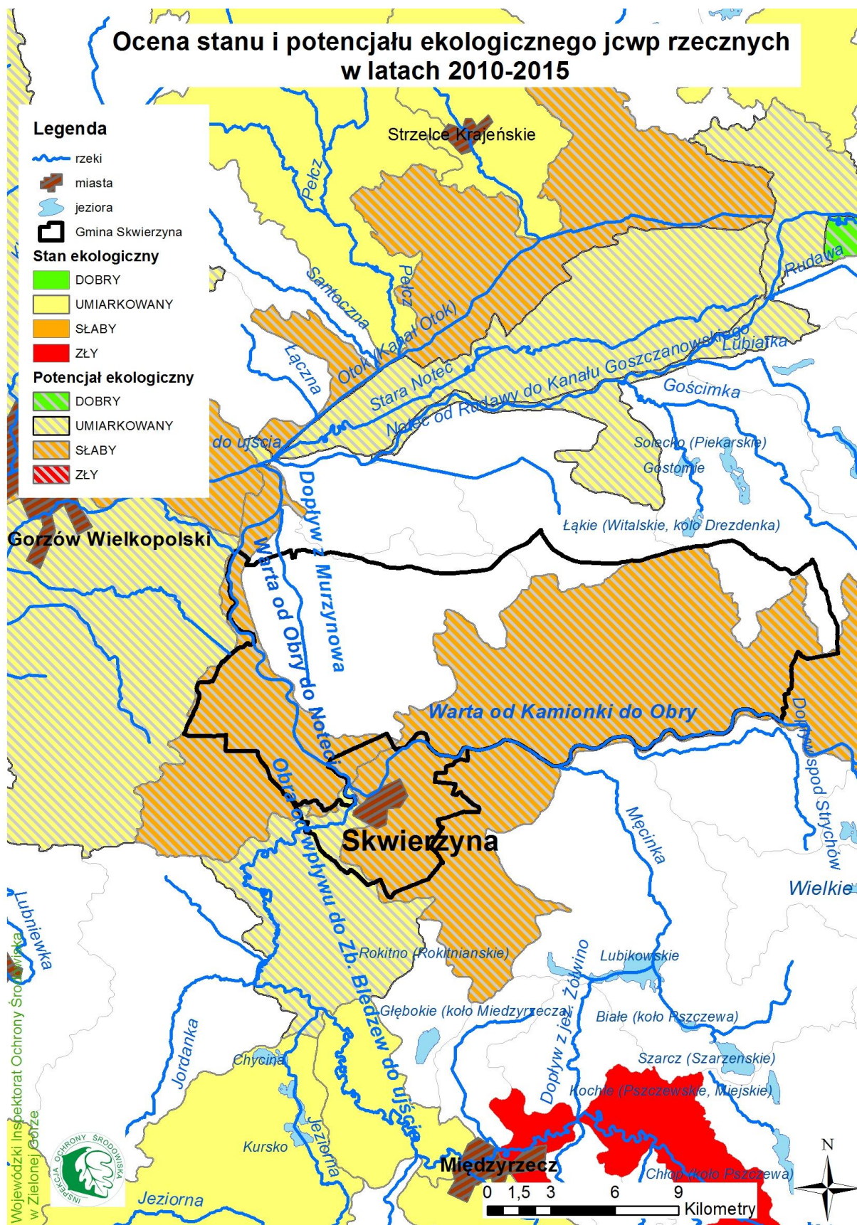
Rys. 6. Ocena stanu i potencjału ekologicznego jcwp rzecznych w Skwierzynie badanych w latach 2010-2015
