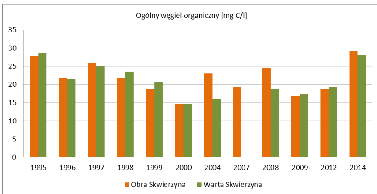
Rys. 13. Średnioroczne wartości stężenia ogólnego węgla organicznego [mg C/l] w wybranych rzekach na terenie Skwierzyny badanych w latach 1995-2014
