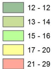
Rys. 35. Rozkład stężeń rocznych pyłu zawieszzonego PM 2,5 w 2016 r. na obszarze gminy Skwierzyna (źródło: GIOŚ)
