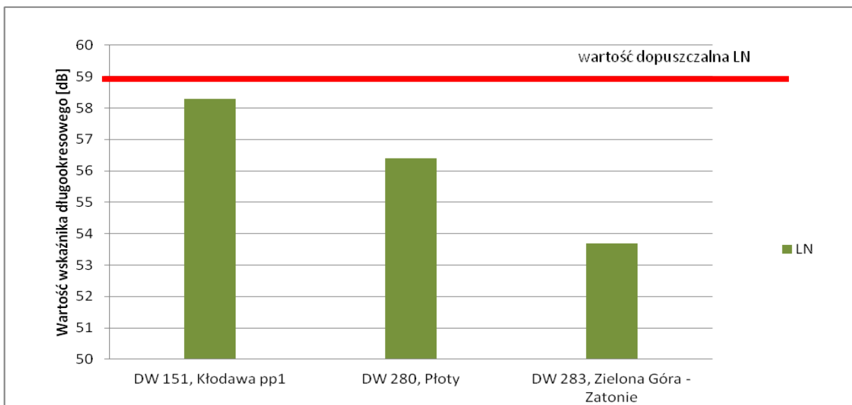
Rys. 40. Wartość zmierzonego poziomu długookresowego L_N w 2016 r. w porównaniu z wartością dopuszczalną
