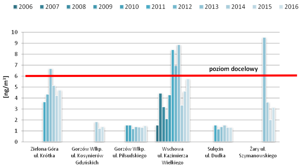
Rys. 30. Wyniki badań stężenia średniorocznego arsenu zawartego w pyłe zawieszonym w powietrzu, wykonanych na obszarze województwa lubuskiego w latach 2006-2016
