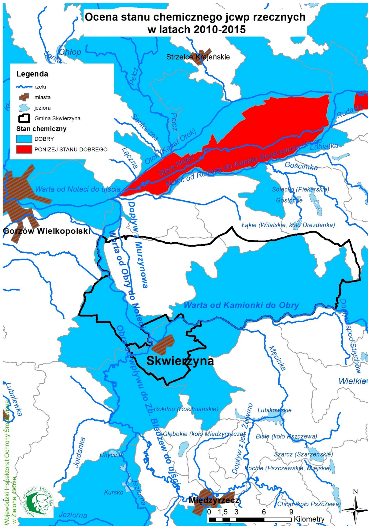
Rys. 7. Ocena stanu chemicznego jcw p rzecznych w Skwierzynie badanych w latach 2010-2015
