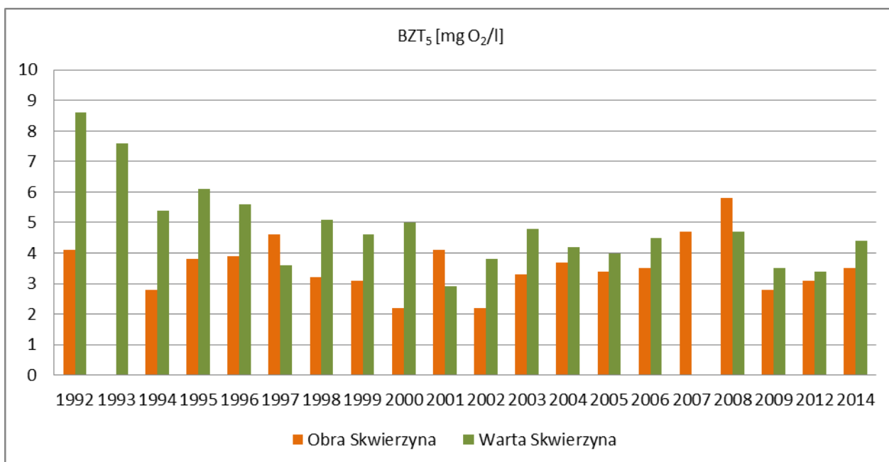
Rys. 12. Średnioroczne wartości BZT 5 [mg O 2 /l] w wybranych rzekach na terenie Skwierzy badanych w latach 1992-2014
