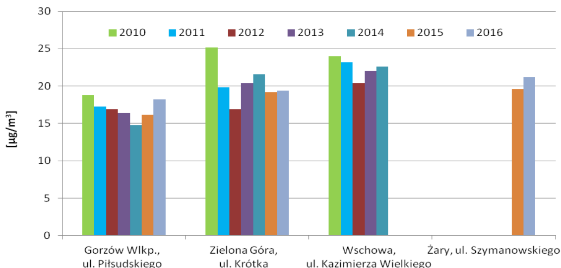
Rys. 28. Wyniki badań stężenia średniorocznego pyłu zawieszonego PM 2,5 w powietrzu, wykonanych na obszarze województwa lubuskiego w latach 2010-2016
