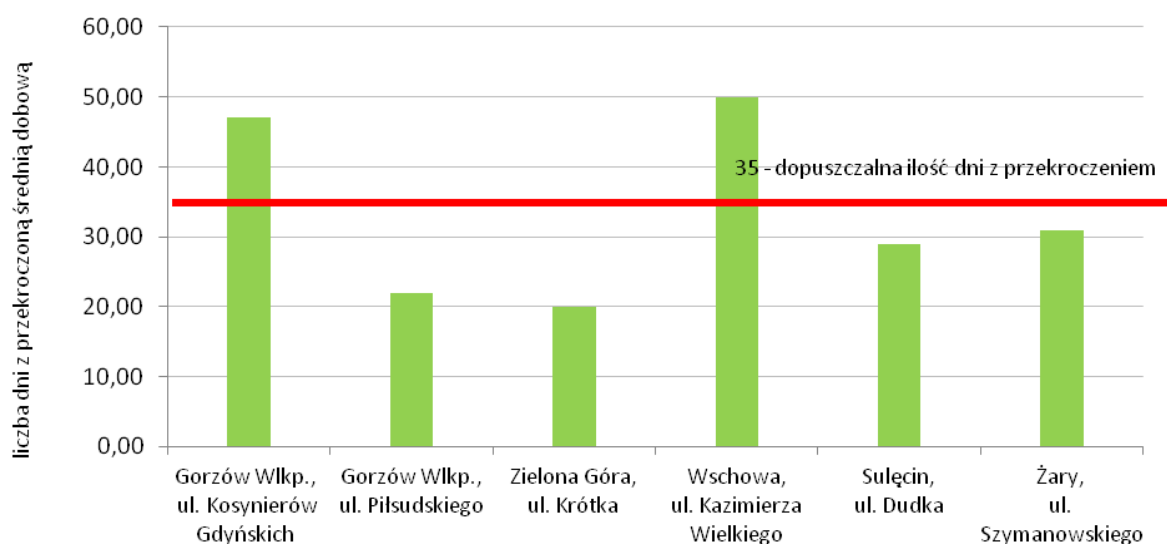
Rys. 24. Liczba dni z przekroczeniem wartości dobowej 50 [\mu\text{g}/\text{m}^3] dla pyłu zawieszzonego PM10 w powietrzu, występujących na obszarze województwa lubuskiego w 2016 roku
