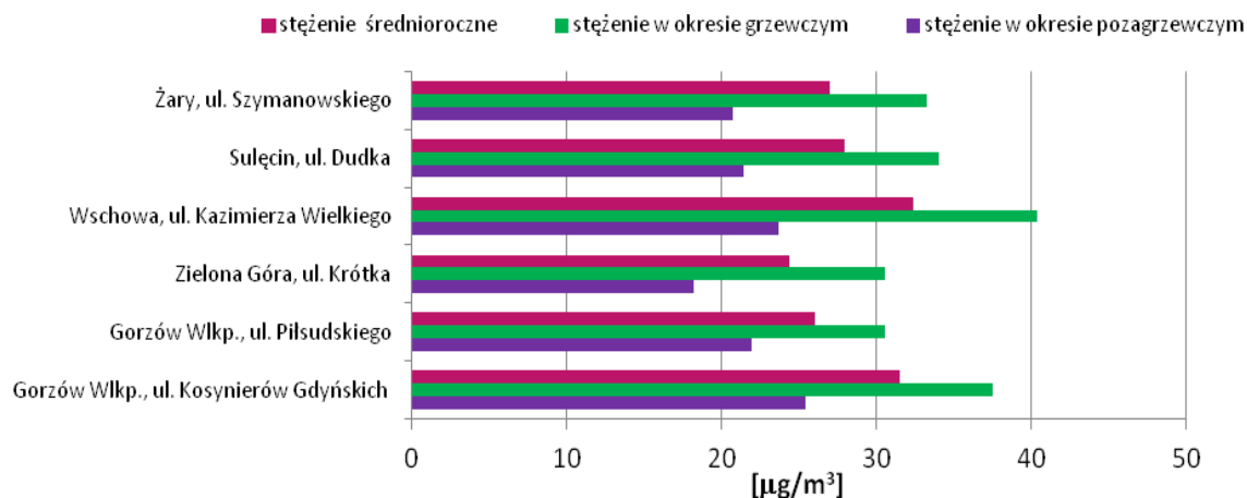
Rys. 23. Wyniki badan stężenia pyłu zawieszzonego PM10 w powietrzu, wykonanych na obszarze województwa lubuskiego w 2016 roku, z podziałem na sezon grzewczy i pozagrzewczy
