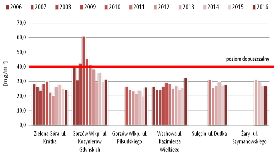
Rys. 22. Wyniki badań stężenia średniorocznego pyłu zawieszonego PM10 w powietrzu, wykonanych na obszarze województwa lubuskiego w latach 2006-2016
