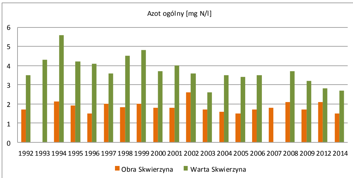
Rys. 9. Średnioroczne wartości stężenia azotu ogólnego [mg N/l] w wybranych rzekach na terenie Skwierzyzny badanych w latach 1992-2014
