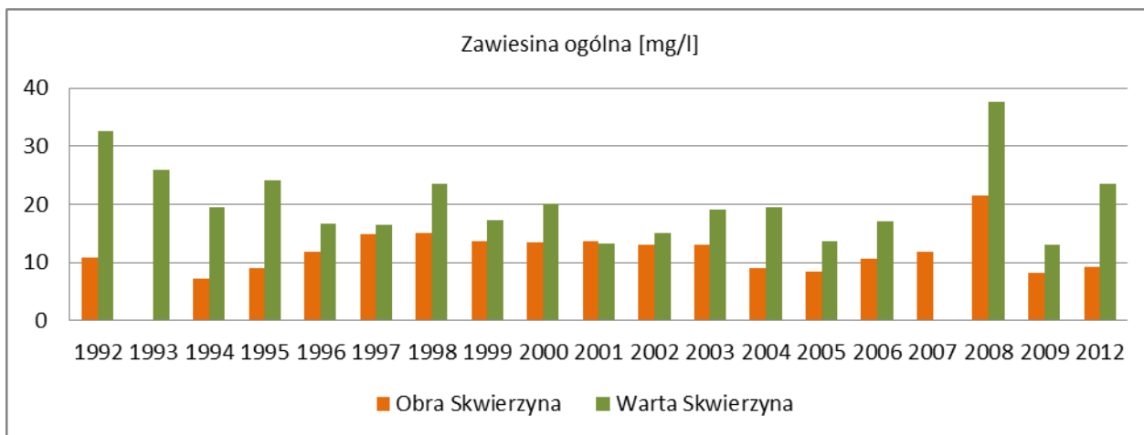
Rys. 11. Średnioroczne wartości stężenia zawiesiny ogólnej [mg/l] w wybranych rzekach na terenie Skwierzy w latach 1992-2012
